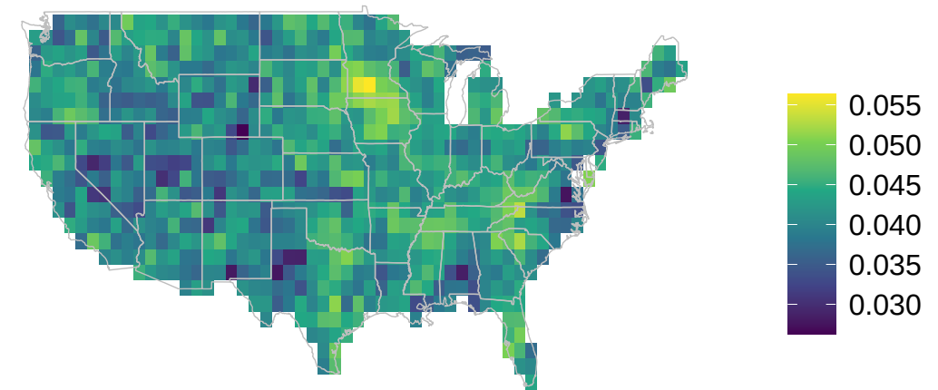
(f) shape parameter uncertainty
