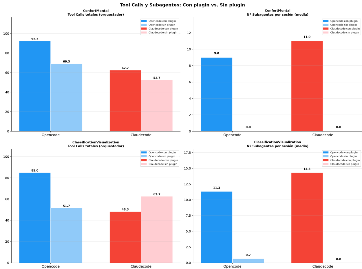
Figura 18: Tool calls totales del orquestador y número de subagentes por sesión, por condición y experimento.
