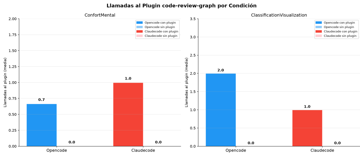
Figura 19: Llamadas al plugin code-review-graph por condición y experimento.
