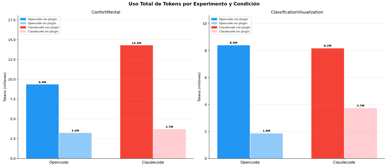
Figura 6: Tokens totales por experimento y condición, separados por asistente. La comparación entre columnas de distinto asistente no es directa por diferencias de tokenizador y caché.
