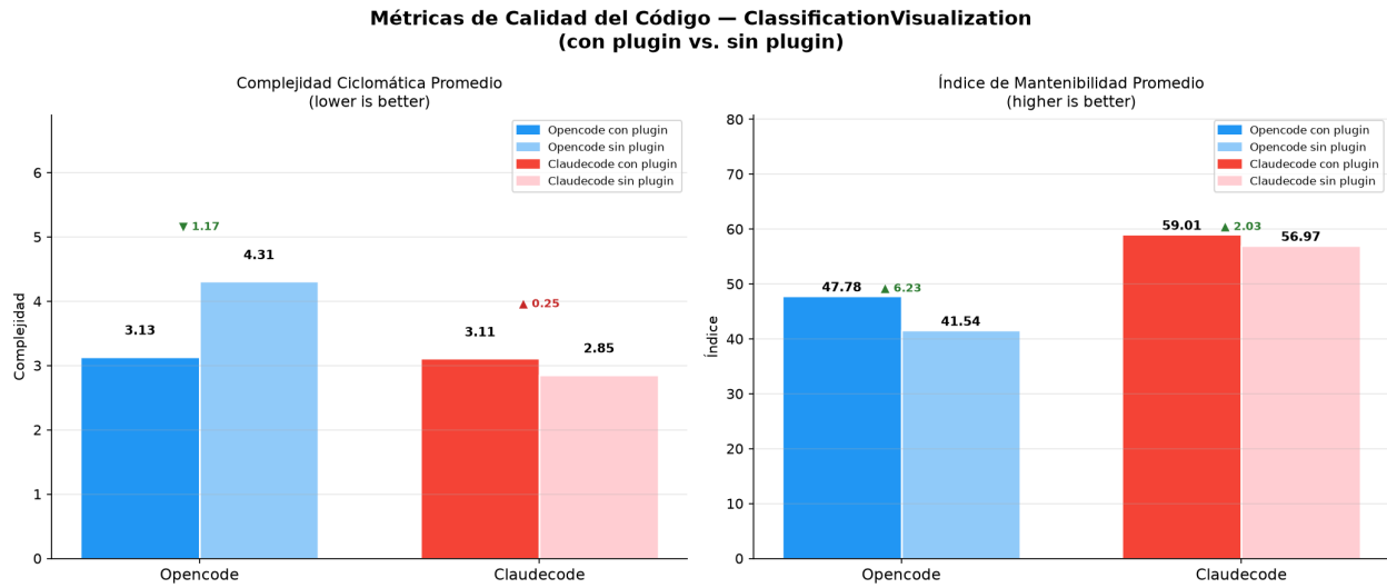
Figura 9: Métricas de calidad del código en el Caso 2 por asistente y condición.
