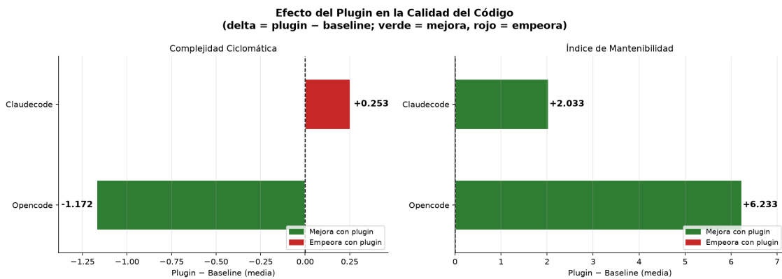
Figura 10: Efecto de colbPowers sobre la calidad del código (delta = colbPowers – baseline). Verde: mejora; rojo: empeora.
