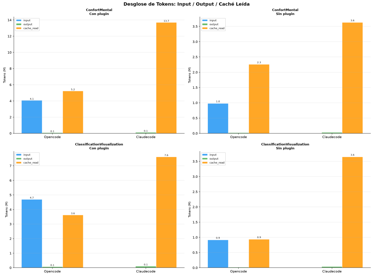
Figura 17: Desglose de tokens por tipo (input, output, caché leída) para cada experimento y condición.
