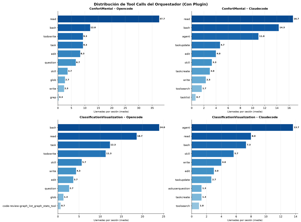
Figura 22: Distribución de tool calls del orquestador por tipo (top 10 herramientas, sesiones con colbPowers).
