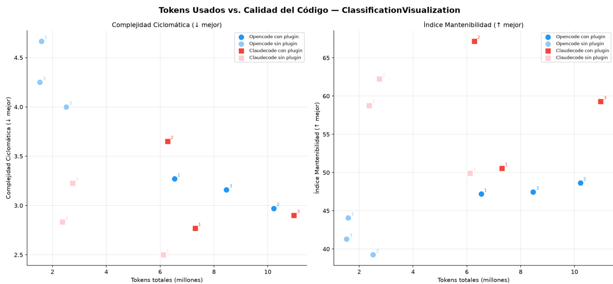
Figura 21: Dispersión: tokens totales vs. métricas de calidad del código (Caso 2). Cada punto representa una sesión individual.
