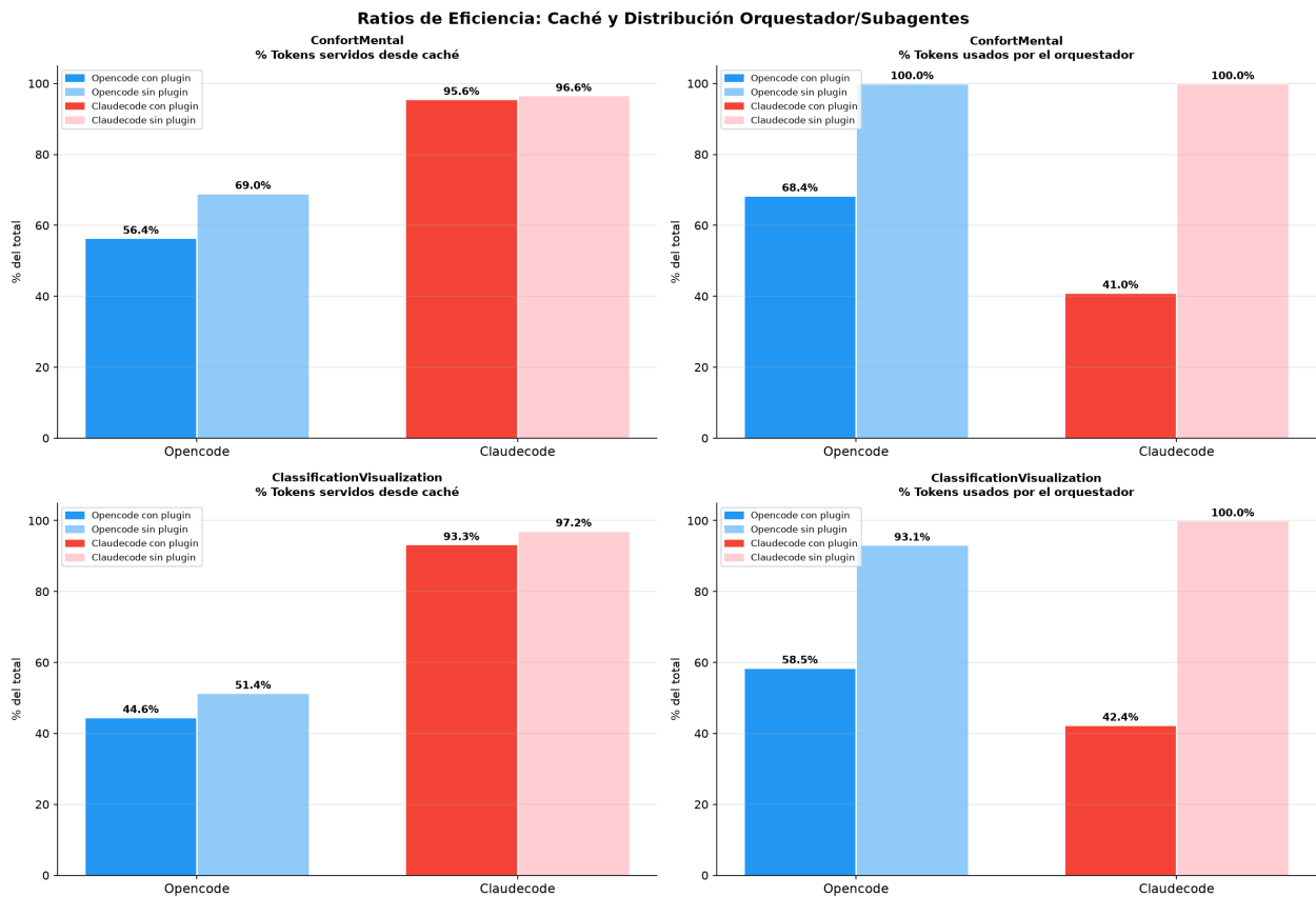
Figura 20: Ratios de eficiencia: porcentaje de tokens servidos desde caché y porcentaje de tokens consumidos por el orquestador.
