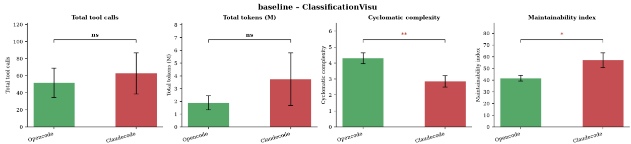
Figura 13: Test t de Welch — OpenCode vs. ClaudeCode, baseline, Caso 2. Los asteriscos indican significancia estadística.
