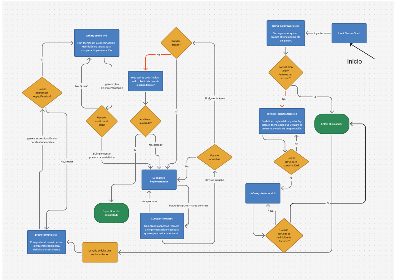
Figura 3: Diagrama de flujo de colbPowers.
