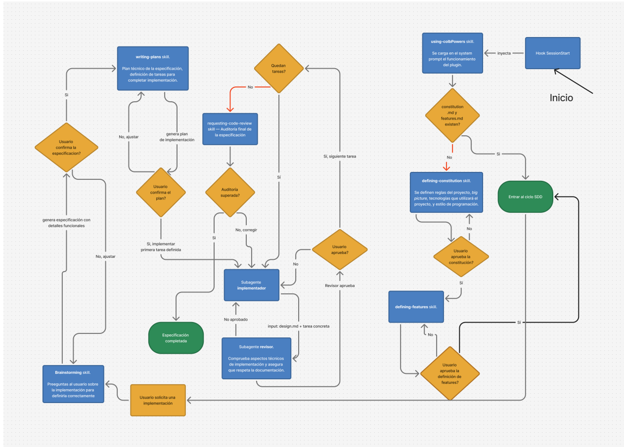
Figura 3: Diagrama de flujo de colbPowers.
