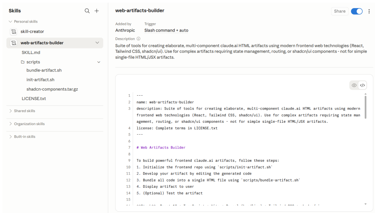
Figura 2: Estructura de una skill en Claude Cowork.
