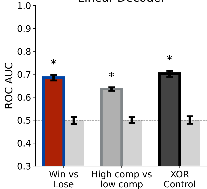
Linear Decoder
