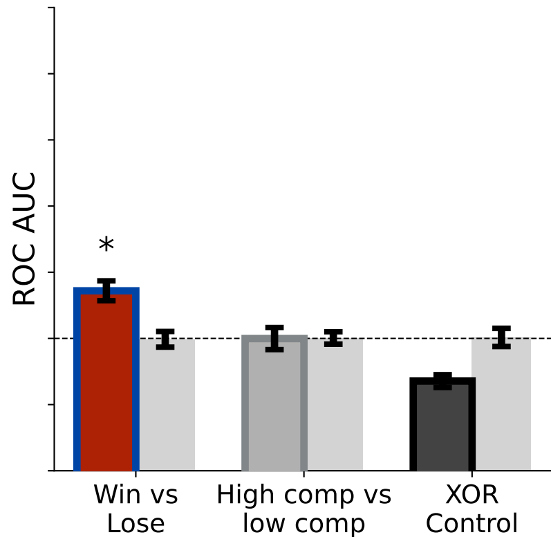
CCGP
