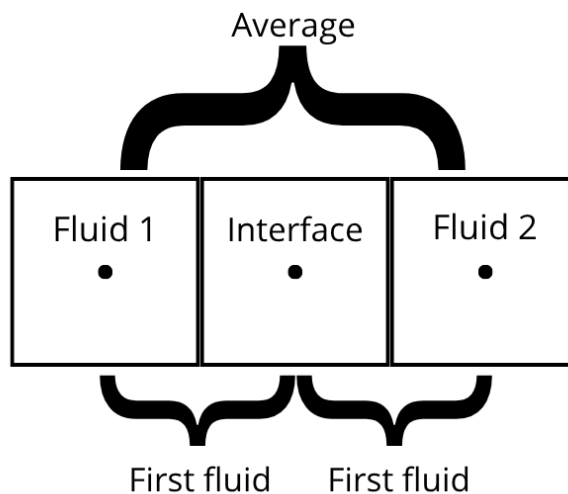
Figura 4.5: Ilustração dos três casos testados para obter a derivada na interface, sendo que as condições são upwind backwind e uma média centrada
