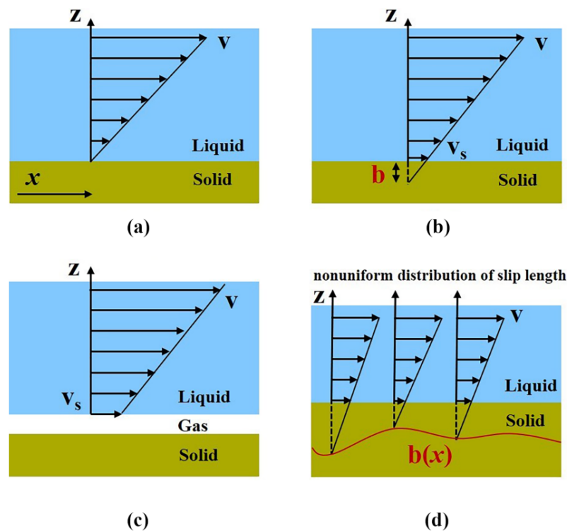
Figura 4.6: Representação do modelo de deslizamento de Navier (Navier-Slip) apresentando o que o comprimento de deslizamento representa. Figura de Wang et al. (2021)
