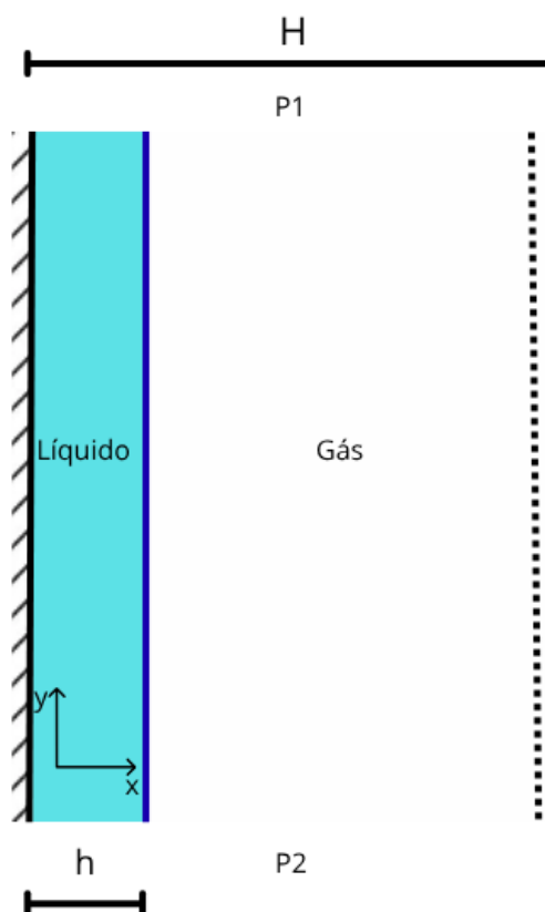
Figura 5.1: Modelo físico do escoamento unidimensional considerado
