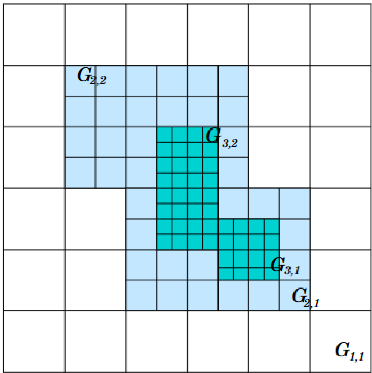
Figura 3.3: Ilustração da hierarquia de níveis utilizada no AMR. Fonte; ?
