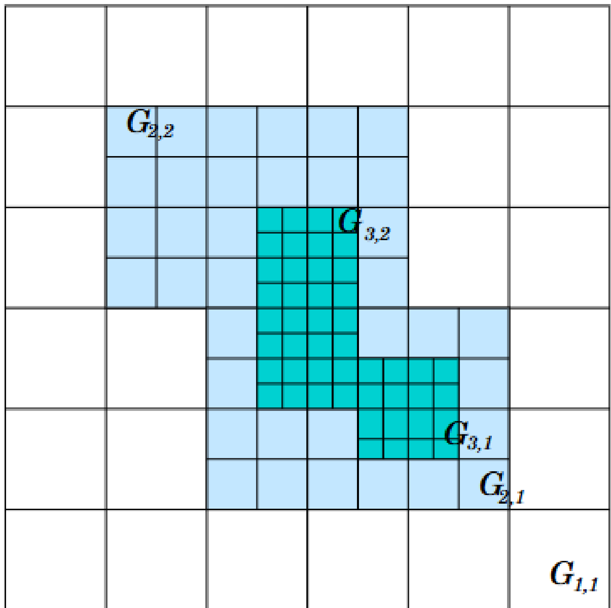
Figura 3.3: Ilustração da hierarquia de níveis utilizada no AMR. Fonte; Villar (2007)
