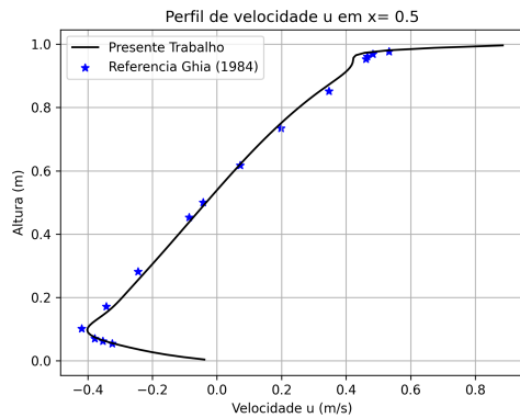
(a) Perfil de velocidade u em x = 0.5 para Re = 3200 .
