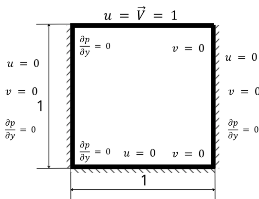
Figura 5.3: Modelo computacional da cavidade com tampa deslizante.
