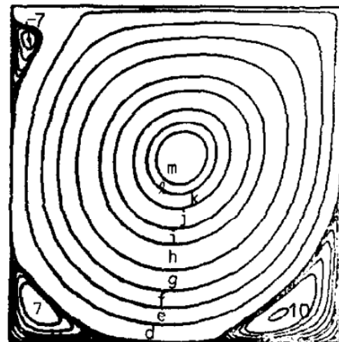
(b) Linhas de fluxo para Re = 3200 . ?
