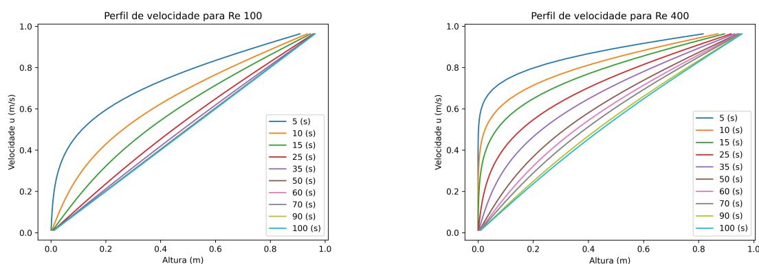
(a) Perfil de velocidade para número de Reynolds 100. Utilizando \nu = 0.01
