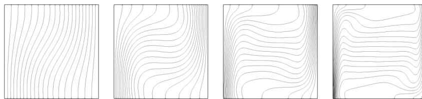
Figura 6.18: Isotermas apresentadas por ?. Da esquerda para a direita o Rayleigh varia de 10^3 a 10^6 em ordem crescente da esquerda para direita.
