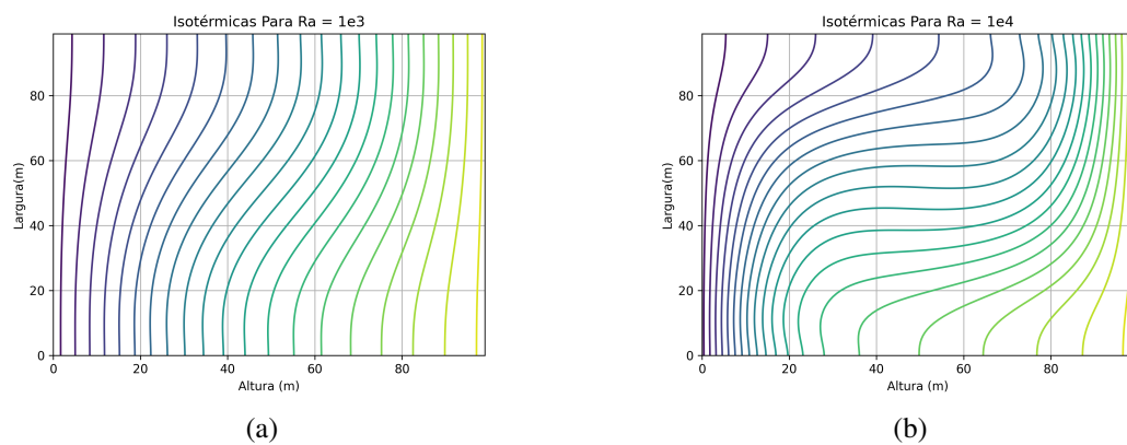
Figura 6.16: Isotermas para números de Rayleigh de 10^3 a 10^4
