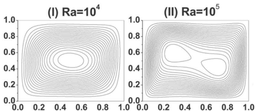
Figura 6.20: Linhas de Fluxo para valores de Rayleigh 10^4 , a esquerda, e 10^5 , a direita. ?.
