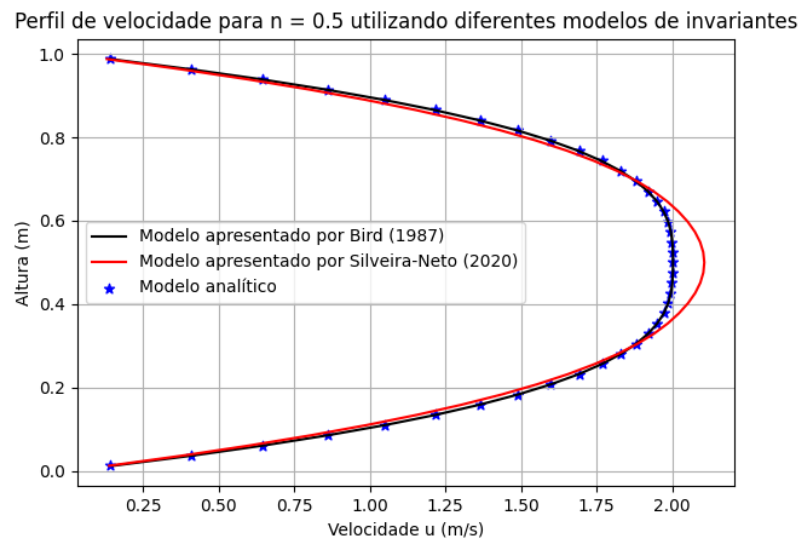
Figura 6.10: Perfis de velocidade para um valor de n = 0.5 e um \Delta p = \sqrt{50} Pa. Comparação do perfil analítico com os invariantes apresentados por ? e ?.
