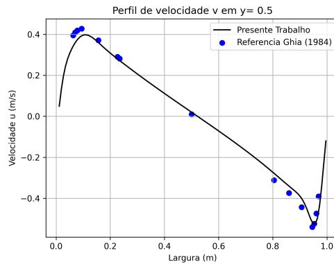
(b) Perfil de velocidade v em y = 0.5 para Re = 3200 .
