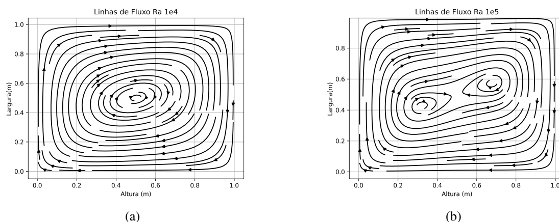
Figura 6.19: Linhas de Fluxo para valores de Rayleigh 10^4 , a esquerda, e 10^5 , a direita.
