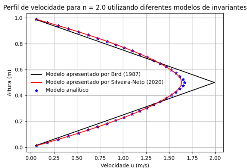
Figura 6.9: Perfis de velocidade para um valor de n = 2 e um \Delta p = 50\text{Pa} . Comparação do perfil analítico com os invariantes apresentados por ? e ?.
