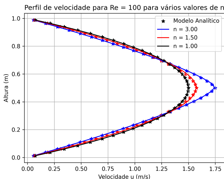
Figura 6.8: Diferentes perfis de velocidade para o escoamento de Poiseuille, com valores de n de 1, 1.5 e 3, para velocidade de entrada constante. Comparação com os resultados do modelo analítico
