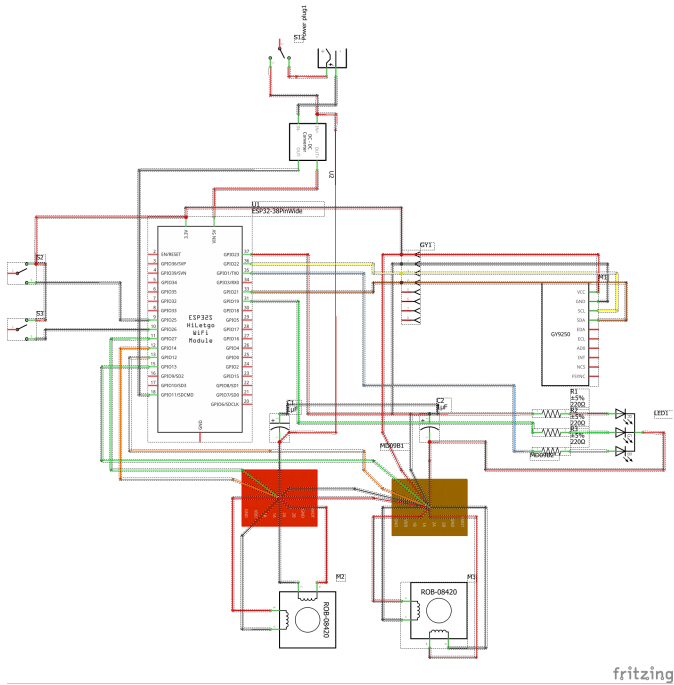
Gambar 3.5 Rangkaian elektronika sistem teleskop
