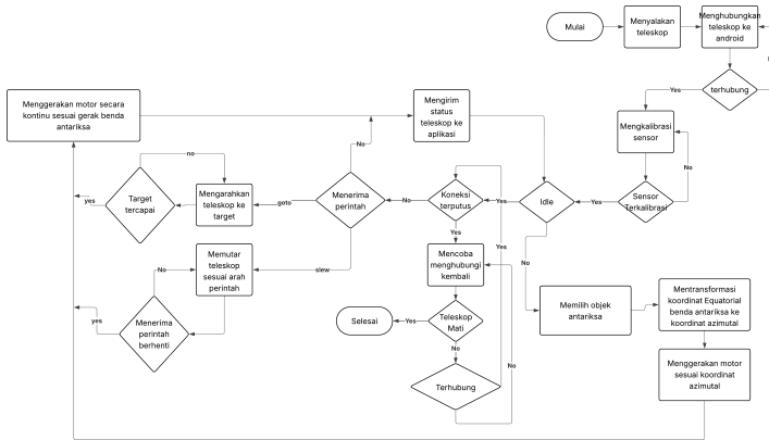
Gambar 3.2 Flowchart sistem kontrol teleskop robotik
