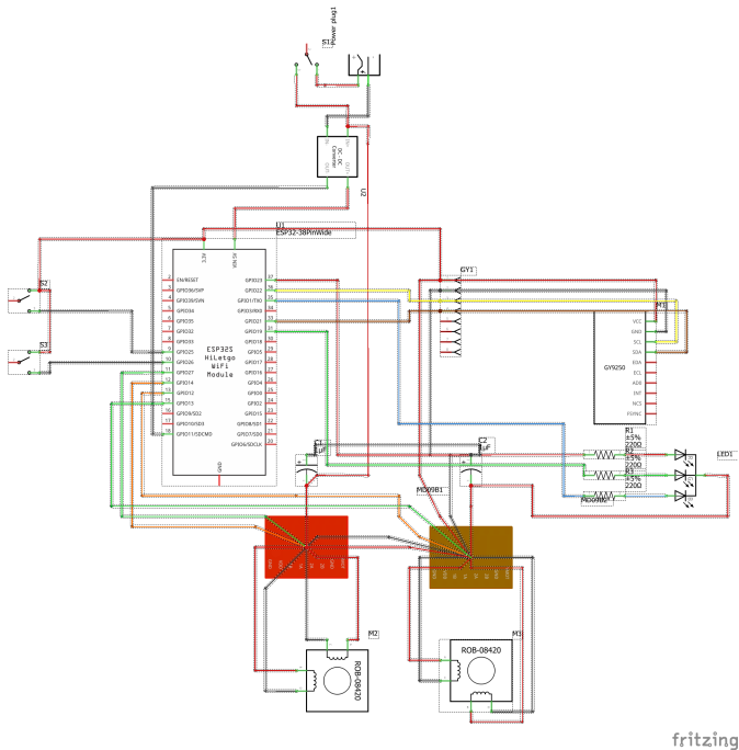
Gambar 3.6 Rangkaian elektronika sistem teleskop
