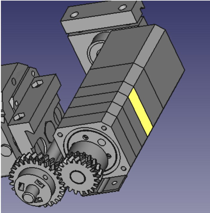
Gambar 3.5 Model 3D planetary gear pada sistem penggerak teleskop
