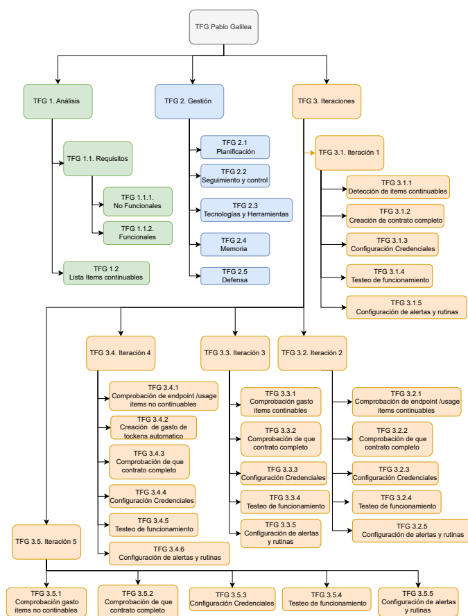
Figura 3.1: EDT
