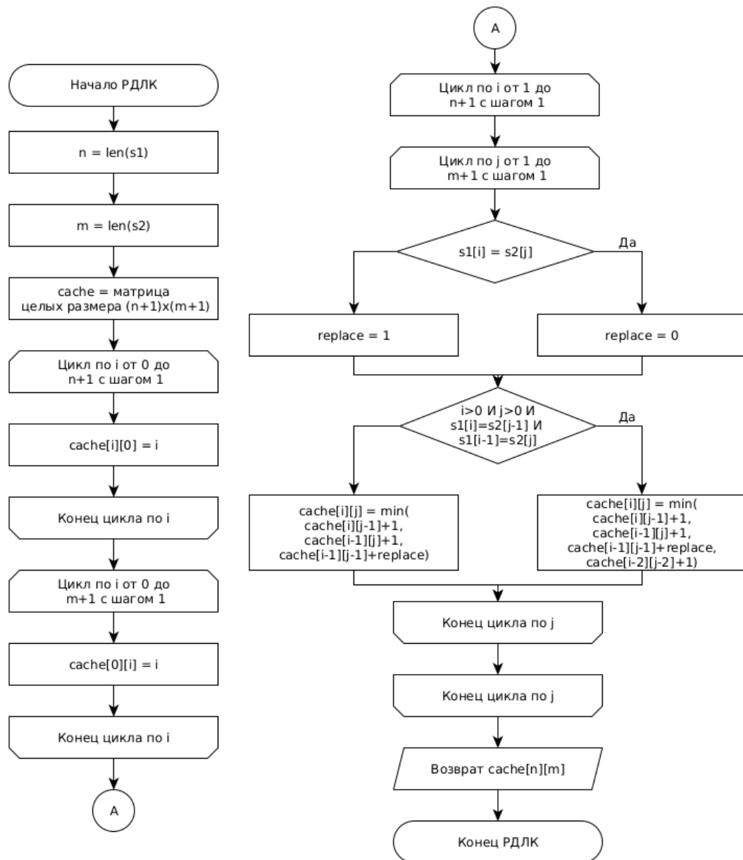
Рисунок 2.3 — Схема алгоритма нахождения расстояния Дамерау-Левенштейна с кешем
