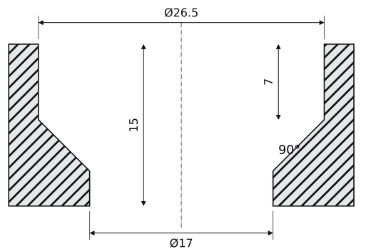
CORTE A-A (2:1)
