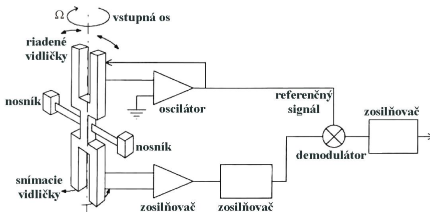
Obr. 3: Principiálna schéma gyroskopu Systron Donner GyroChip [6]
