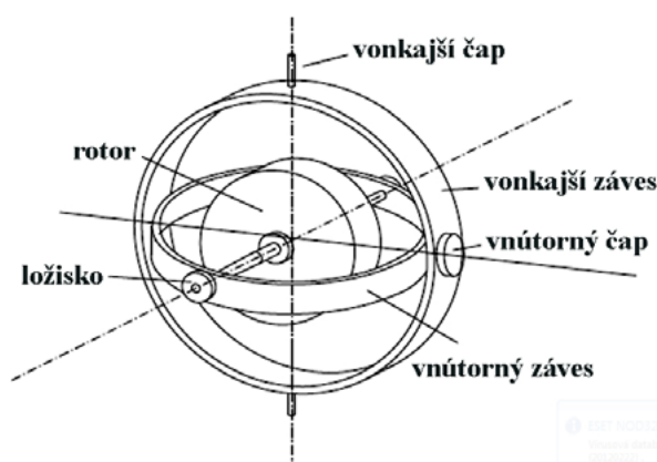
(b) Dvojosý mechanický gyroskop so zotrvačníkom [6]
