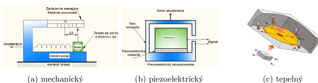
Obr. 4: Štruktúra a princíp merania rôznych typov akcelerometrov [6]
