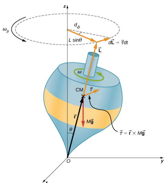
(a) Precesia gyroskopu so znázornením všetkých pôsobiacich síl a momentov [15]
