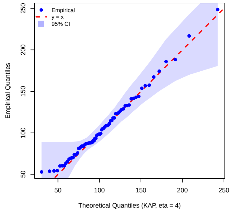
Kappa Q-Q Plot (eta = 4 )
