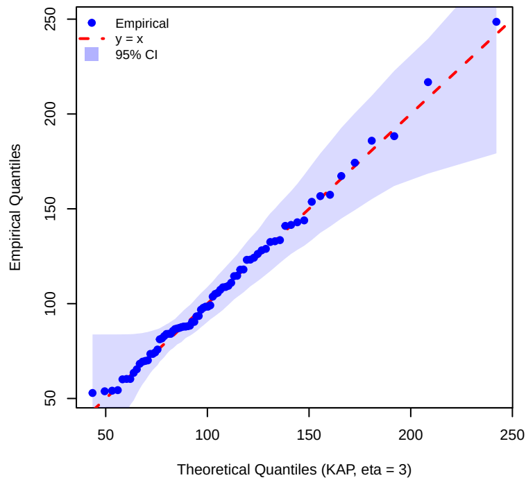
Kappa Q-Q Plot (eta = 3 )
