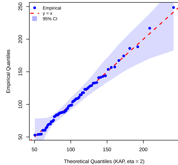
Kappa Q-Q Plot (eta = 2 )
