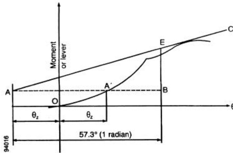
그림 2. 동복원력 곡선
