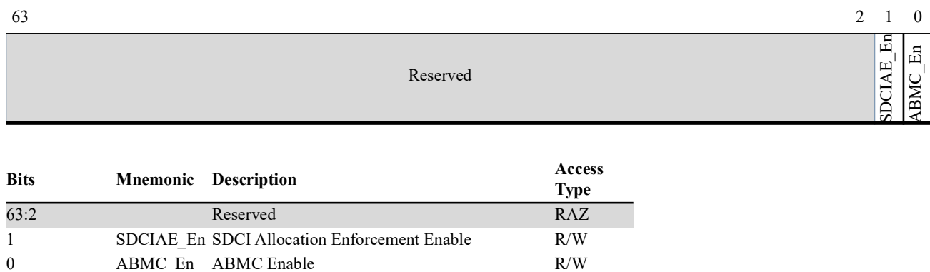
Figure 19-7. L3_QOS_EXT_CFG
