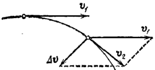
Рис. 6: Изменение скорости
