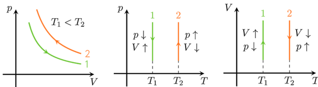
Рис. 3: Графики изотермического процесса
