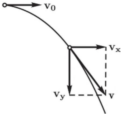
Рис. 6: Разложение скорости на проекции
