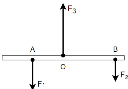
Рис. 11: Равновесие тела при трех параллельных силах
