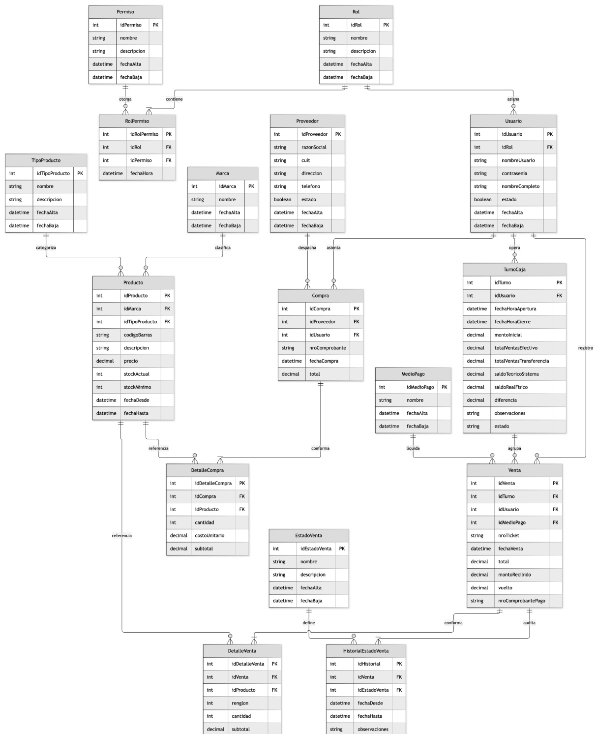
Figura 18: Diagrama de Entidad-Relación general.
