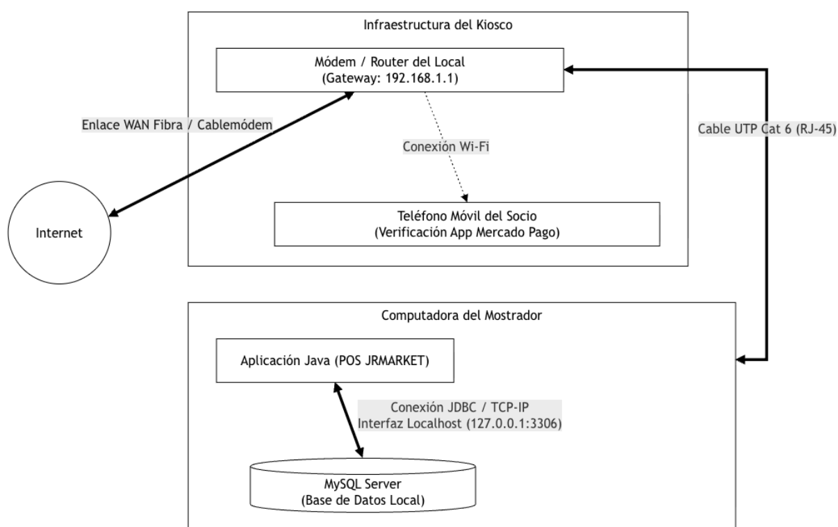
Figura 5: Diagrama de Comunicaciones y Conectividad Local.
