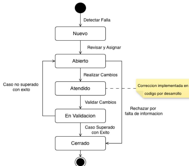
Figura 16: Diagrama de Estados de tratamiento de defectos.
