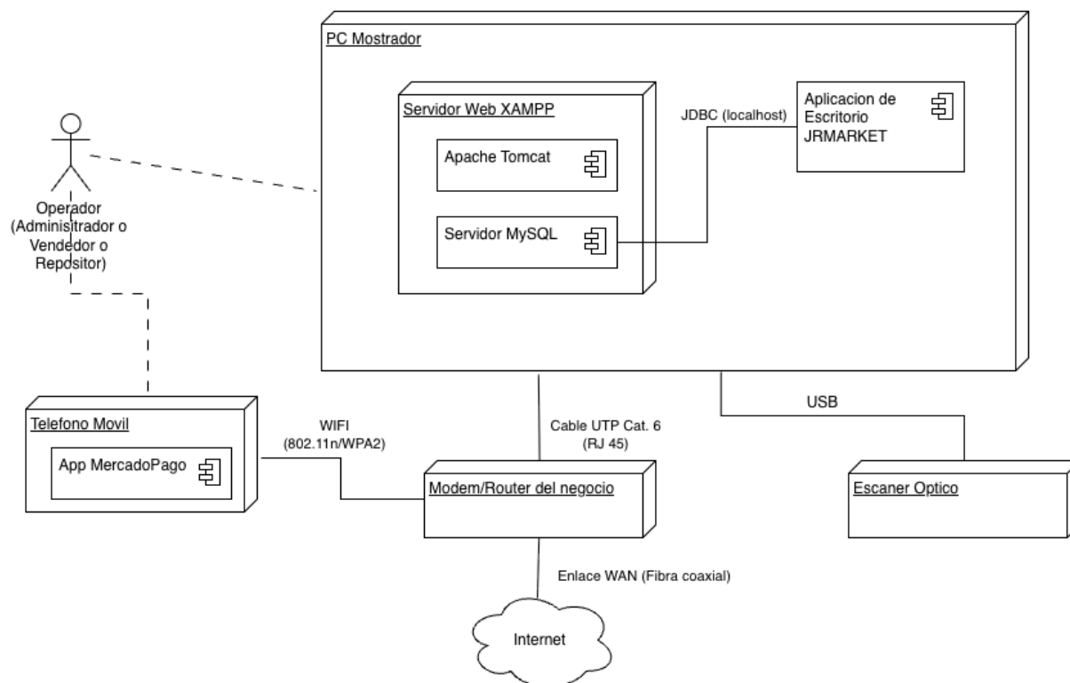
Figura 16: Diagrama de Componentes del Sistema.
