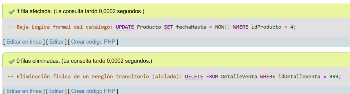
Figura 28: Resultado de ejecución de operación Update y Delete desde phpMyAdmin.
