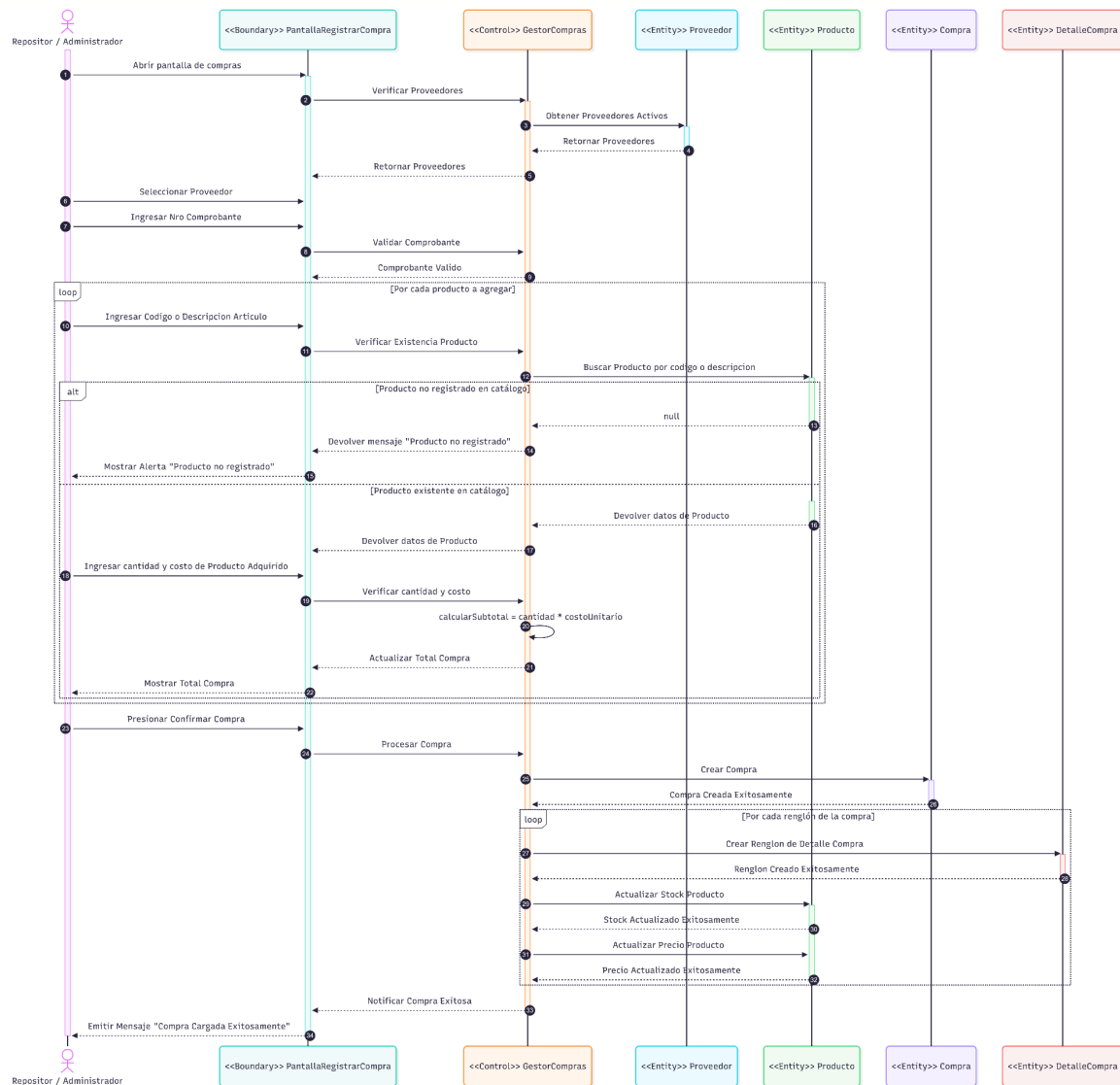
Figura 14: Diagrama de Secuencia del Análisis - Compra de Productos.
