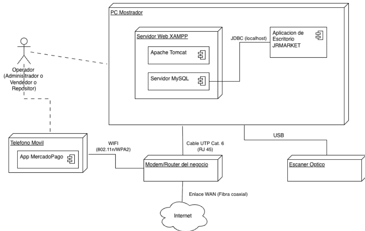
Figura 16: Diagrama de Despliegue del Sistema.
