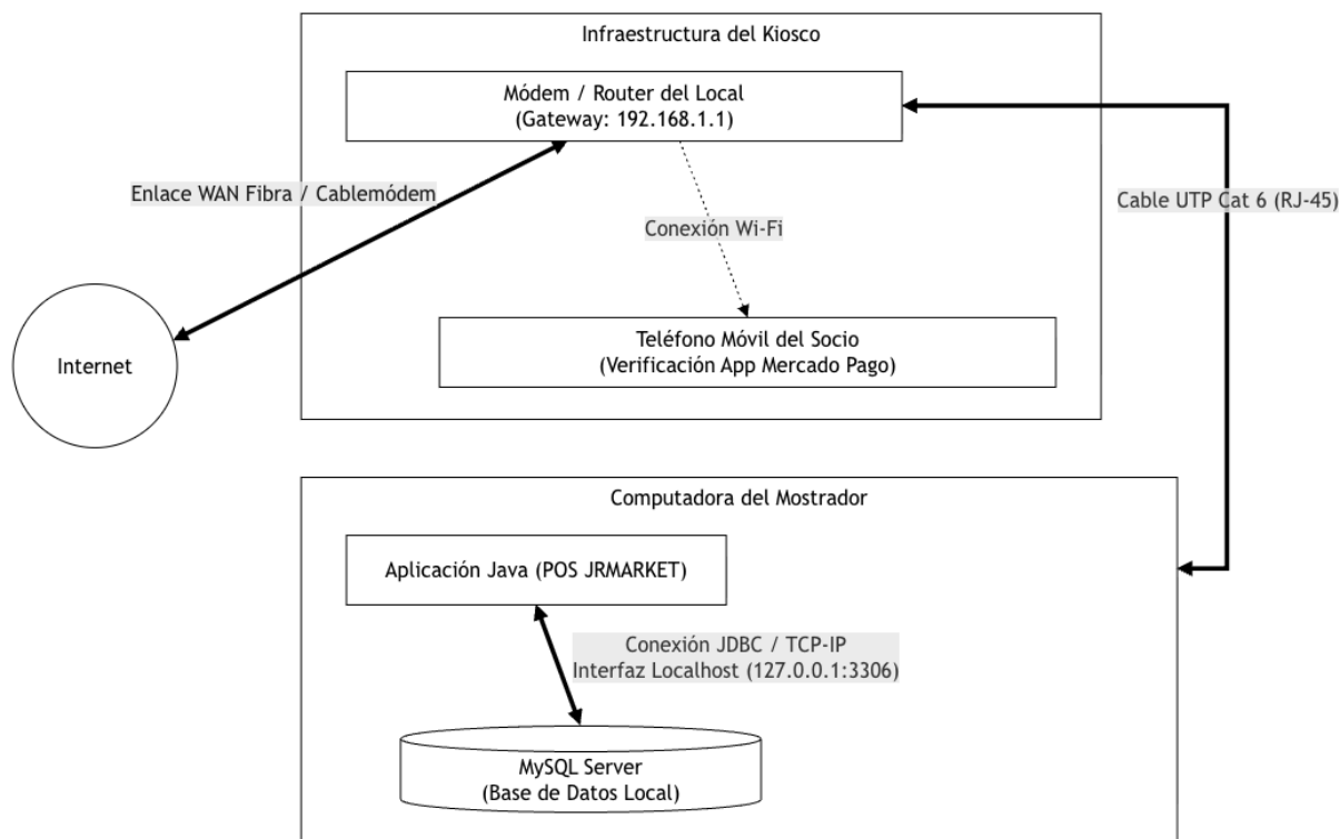
Figura 6: Diagrama de Comunicaciones y Conectividad Local.
