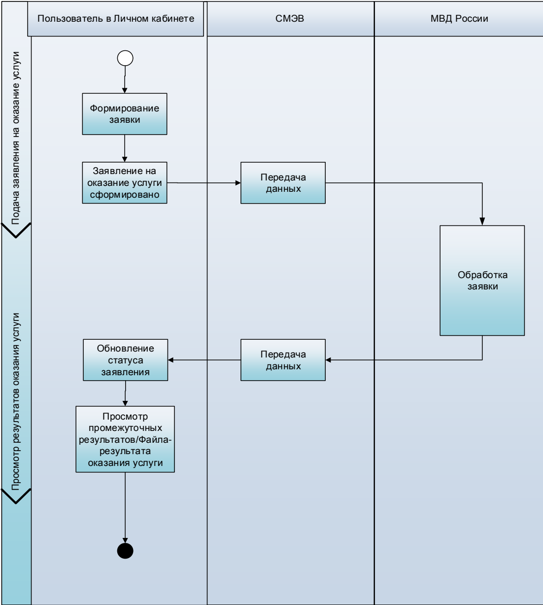
Рисунок 2 – Общий процесс обработки заявления на оказание государственной услуги
