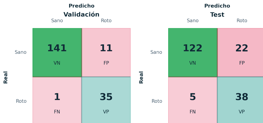
Figura 3.4: Matrices de confusión del ensemble ResNet50 en validación (izquierda) y test (derecha), con el umbral clínico fijado en validación.
