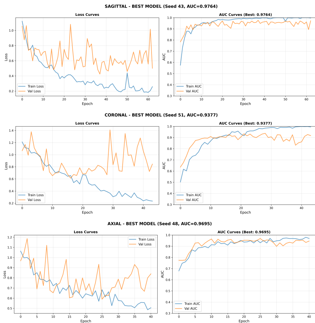
Figura 3.8: Curvas de entrenamiento de los mejores checkpoints de ViT-Small por plano anatómico.
