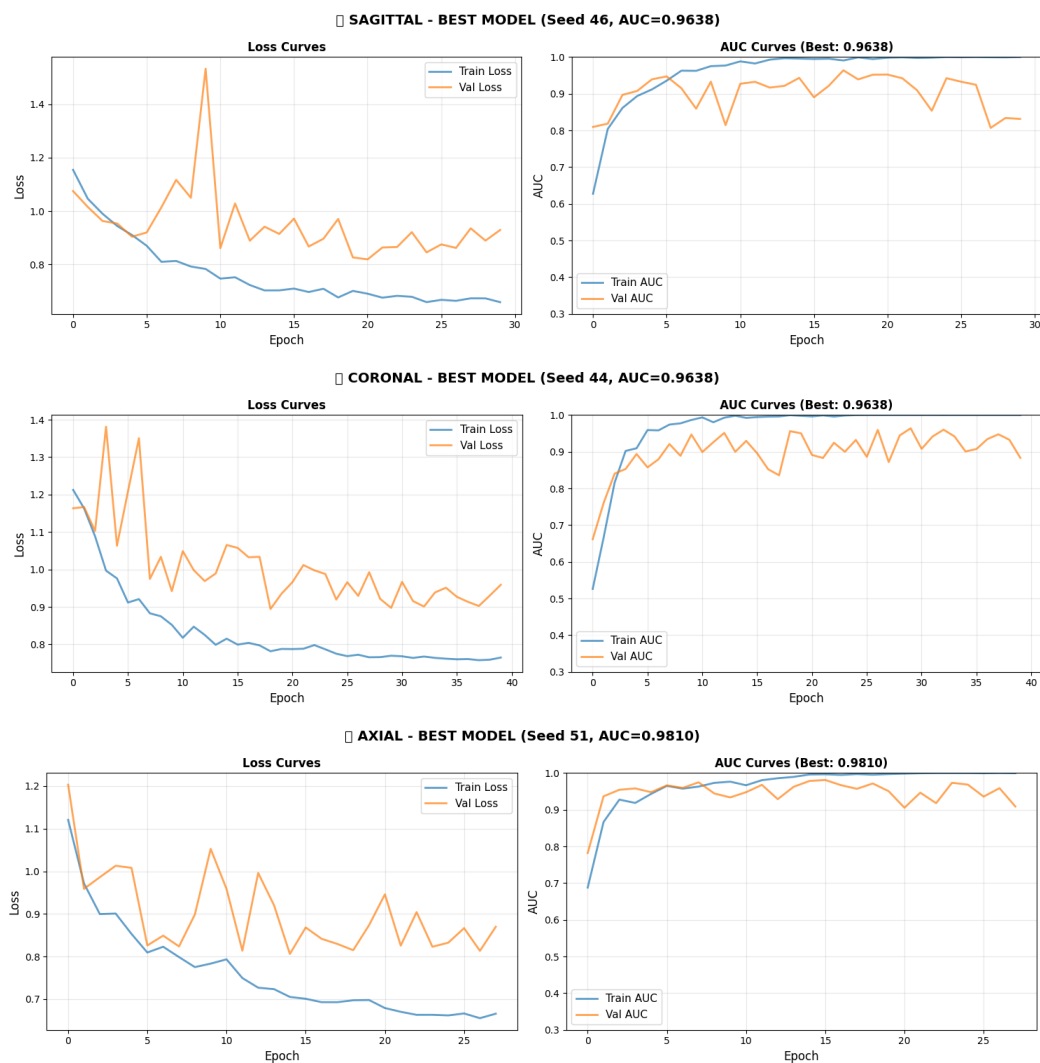
Figura 3.3: Curvas de entrenamiento de los mejores checkpoints de ResNet50 por plano anatómico.
