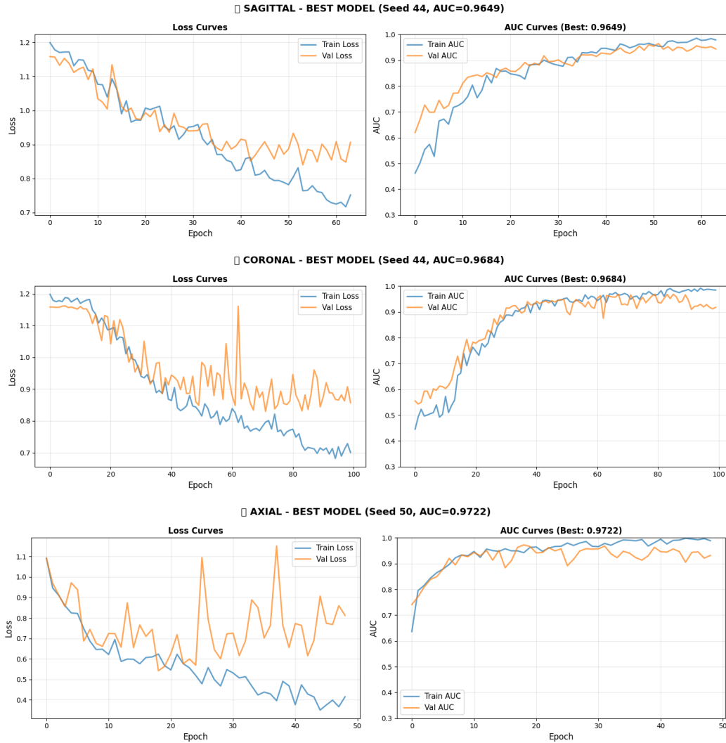
Figura 3.11: Curvas de entrenamiento de los mejores checkpoints de Swin-Tiny por plano anatómico.
