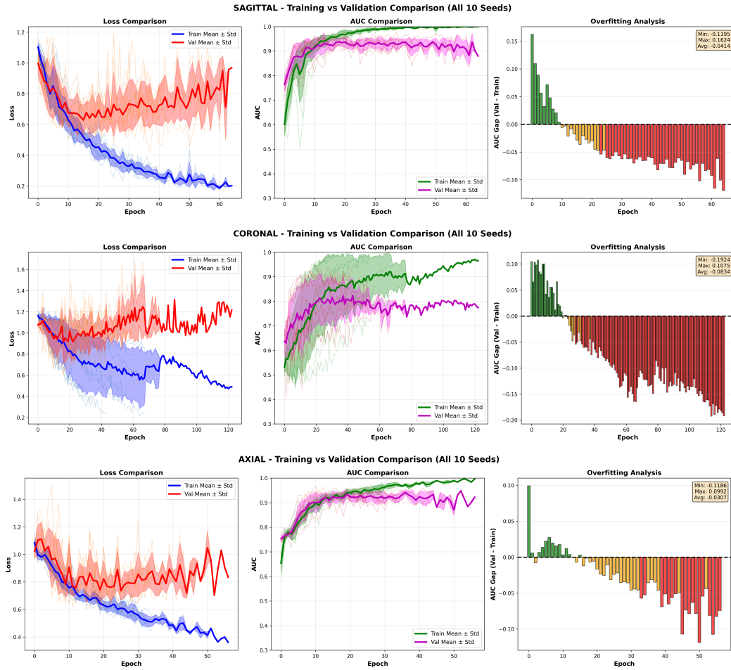
Figura 3.6: Evolución del entrenamiento multi-semilla de ViT-Small en los planos sagital, coronal y axial. Cada figura recoge, de izquierda a derecha, la pérdida de entrenamiento y de validación, el AUC de entrenamiento y de validación, y el análisis de sobreajuste —la brecha de AUC entre validación y entrenamiento (Val – Train) en cada época—; las curvas representan la media \pm desviación típica de las diez semillas.
