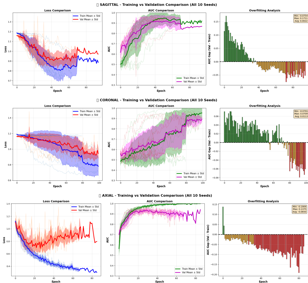
Figura 3.10: Evolución del entrenamiento multi-semilla de Swin-Tiny en los planos sagital, coronal y axial. Cada figura recoge, de izquierda a derecha, la pérdida de entrenamiento y de validación, el AUC de entrenamiento y de validación, y el análisis de sobreajuste —la brecha de AUC entre validación y entrenamiento (Val – Train) en cada época—; las curvas representan la media \pm desviación típica de las diez semillas.
