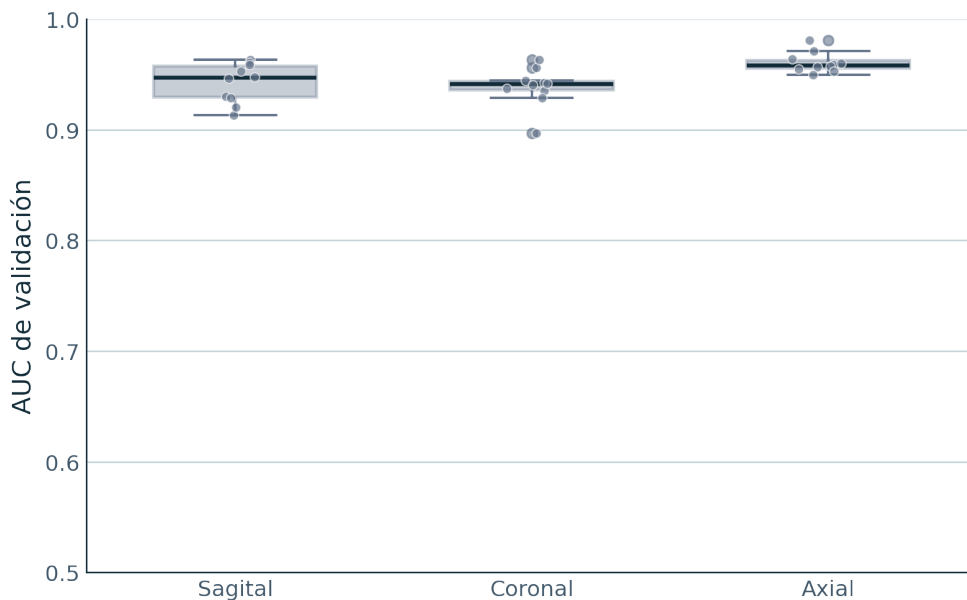
Figura 3.1: Distribución del AUC de validación de ResNet50 sobre las diez semillas (42–51) en cada plano anatómico. Cada punto corresponde a una semilla; la caja representa el rango intercuartílico y la línea central, la mediana.
