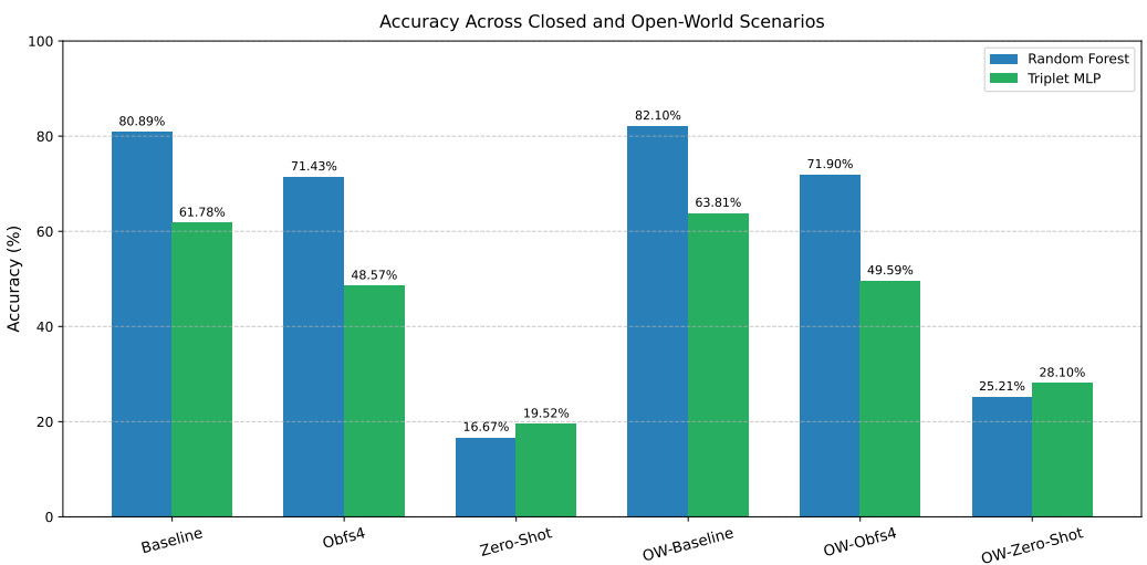
4. ábra. Pontosság alakulása minden beállításban, zárt és nyílt világú esetekben.
