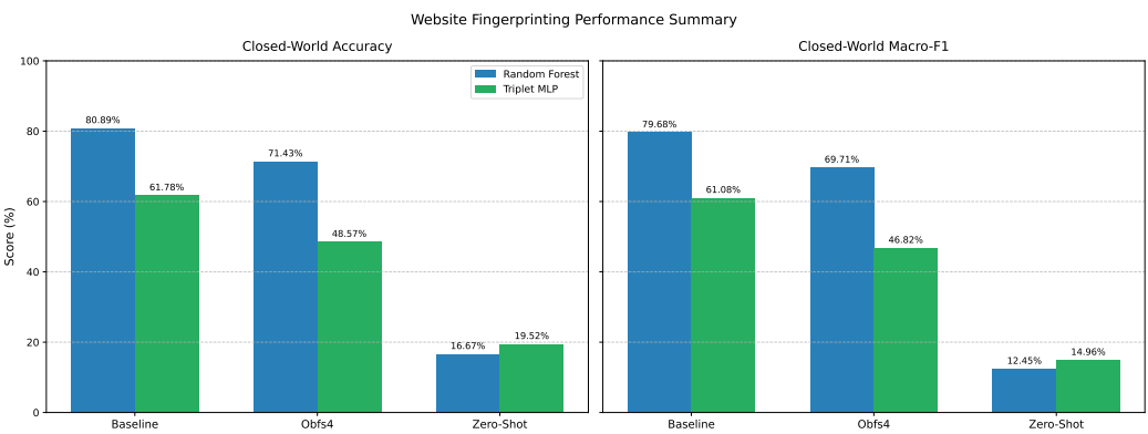
2. ábra. Zárt világú teljesítmény-összegzés (pontosság és macro-F1) a két modellre.
