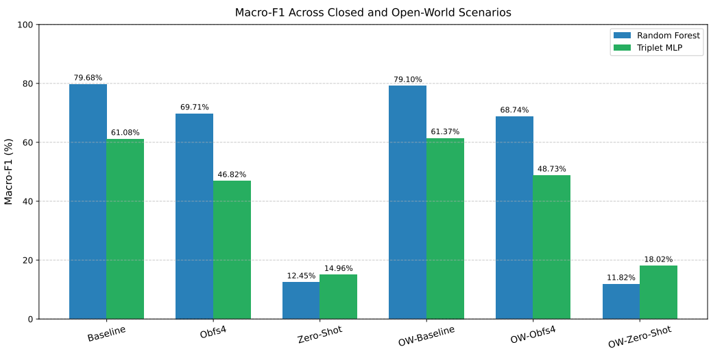
3. ábra. Macro-F1 alakulása minden beállításban, zárt és nyílt világú esetekben.
