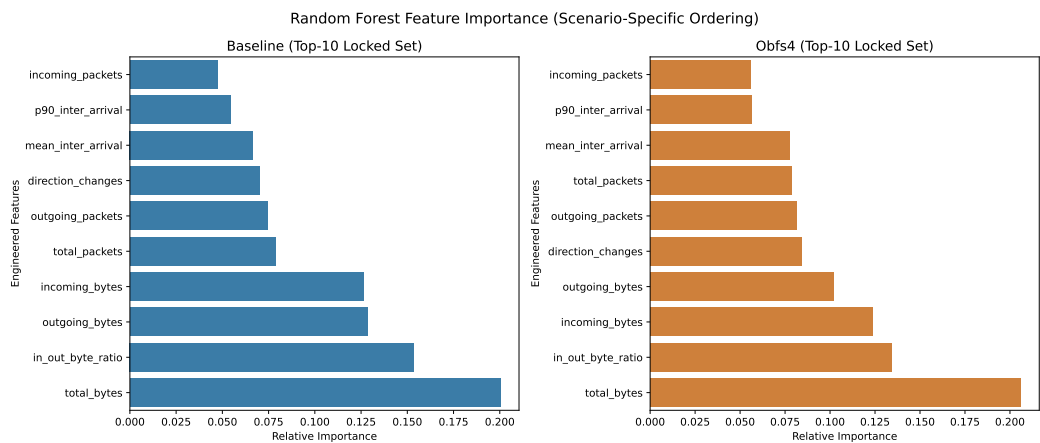
7. ábra. A top-10 jellemzők fontossága a közös (shared) kiválasztás mellett.
