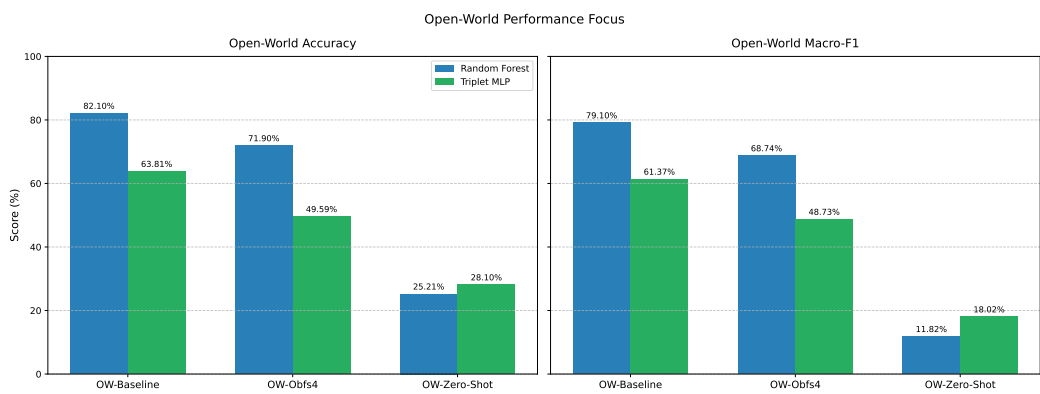
6. ábra. Nyílt világú beállítások összehasonlítása.
