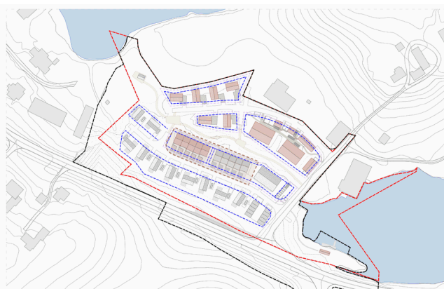
Oversiktsplan 1:2000
