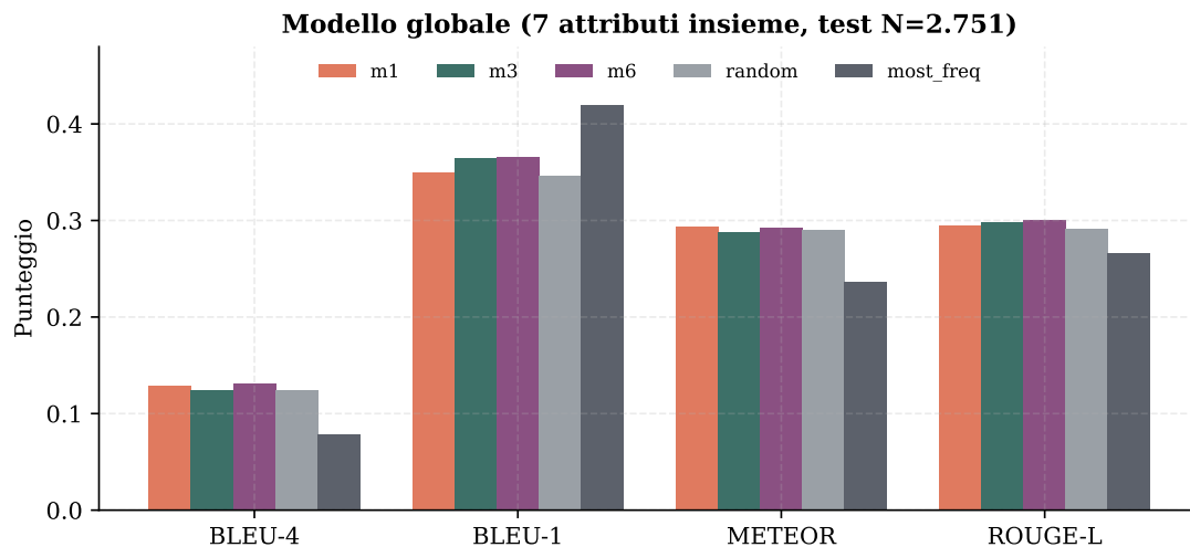
Figura 13: Modello globale (7 attributi insieme). m6 vince di misura su BLEU-4, BLEU-1 e ROUGE-L; i tre modelli restano in un cluster strettissimo (spread 0,007 BLEU-4). Nota: most_frequent ha il BLEU-1 più alto ma il BLEU-4 peggiore — comportamento degenerare “predici sempre la maggioranza”.
