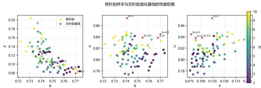
图 4: 热阻、压降与温度非均匀性之间的性能权衡。圆点为有针肋样本, 星形为相同歧管深高比下的无针肋基线。
