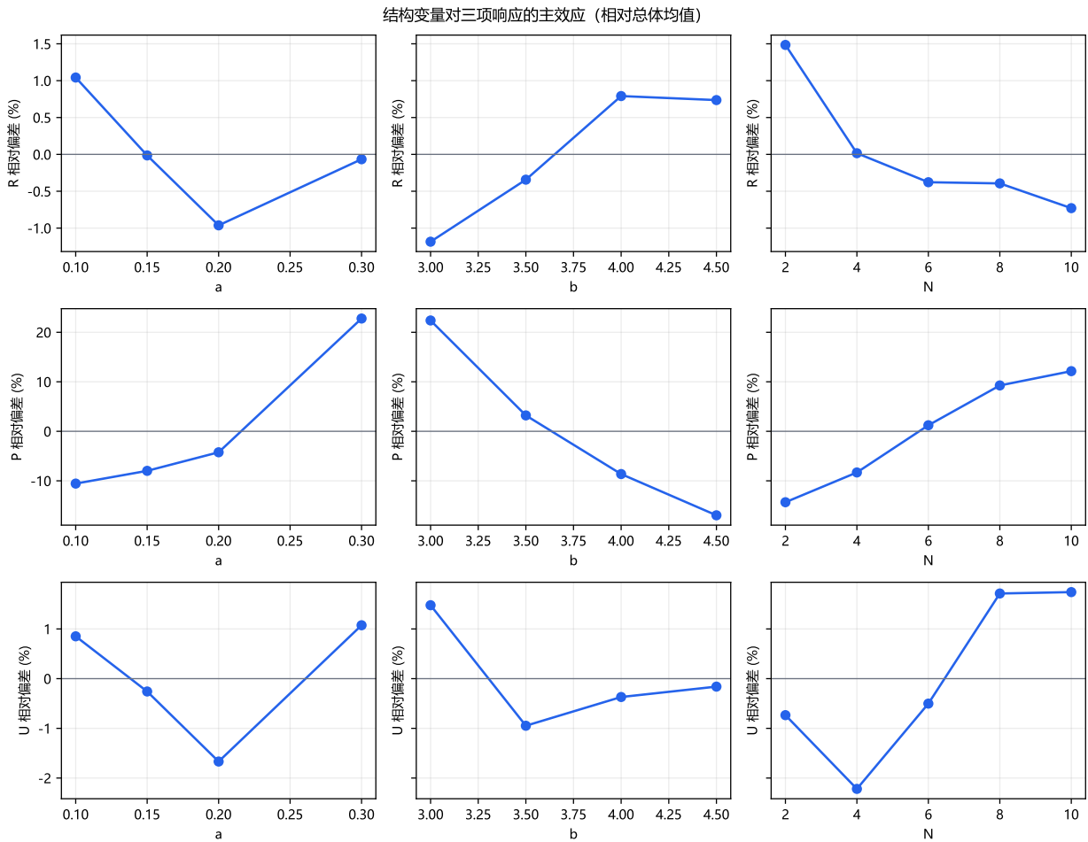
图 3: 三个结构参数对系统性能指标的主效应。三项指标均越小越优；边际均值表示其他参数取各水平时的平均表现。
