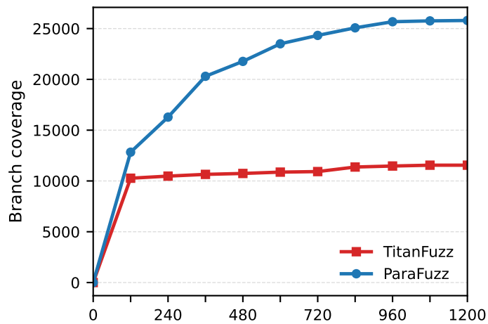
PyTorch vs. TitanFuzz
