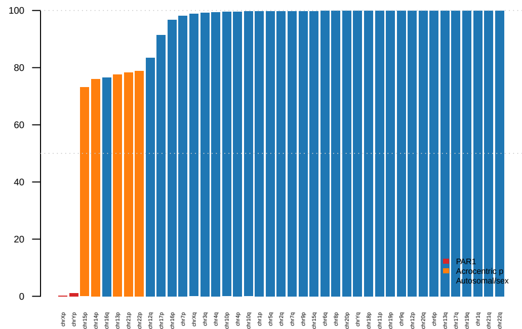
a TAR1 prevalence per arm (n=41)
