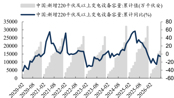
图43: 新增 220kV 及以上变电容量累计 (左轴: 累计值-万千伏安; 右轴: 累计同比)
