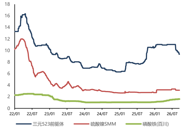
图23: 前驱体价格走势 (万元/吨)
