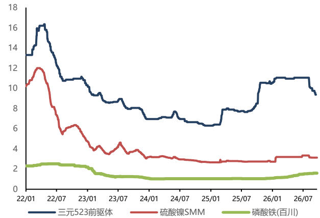
图26: 前驱体价格走势 (万元/吨)
