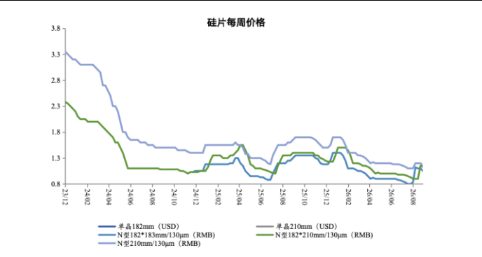
图35：硅片价格走势（元/片）
