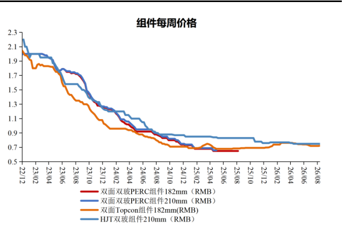
图37：组件价格走势（元/W）
