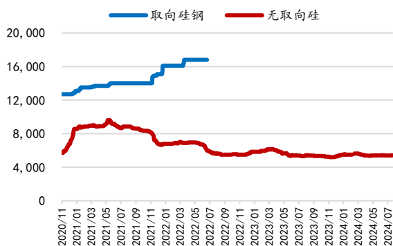
图48: 取向、无取向硅钢价格走势（元/吨）
