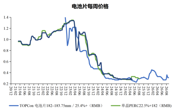
图36: 电池片价格走势 (元/W)
