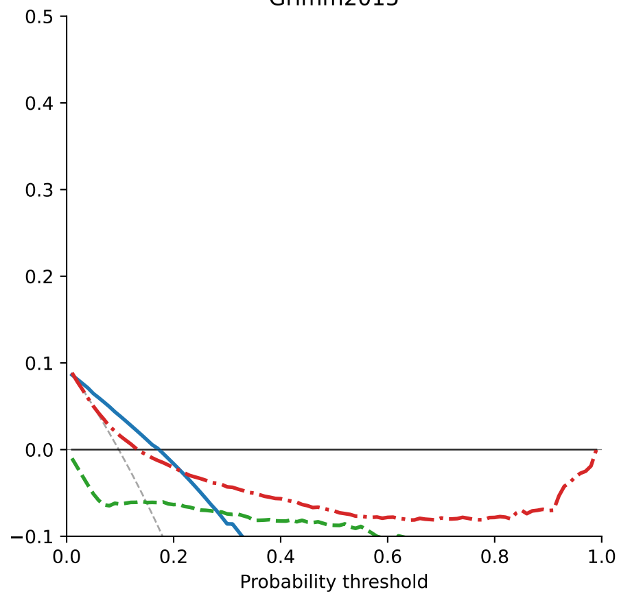
Grimm2015
