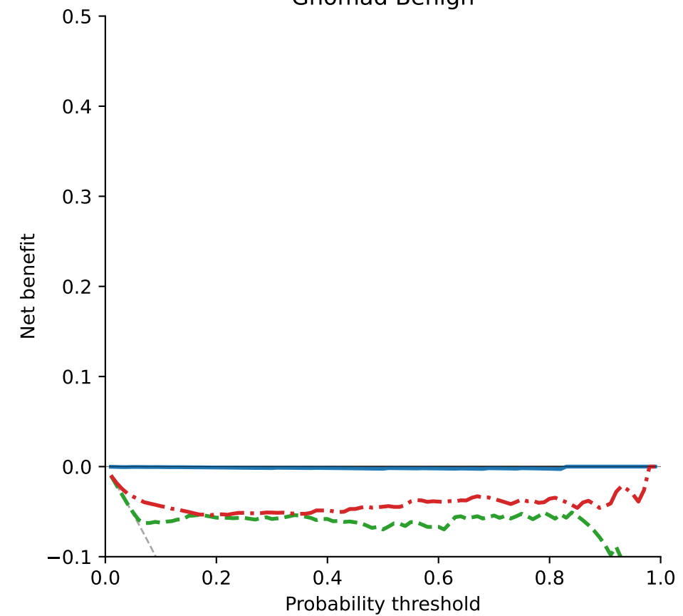
Gnomad Benign
