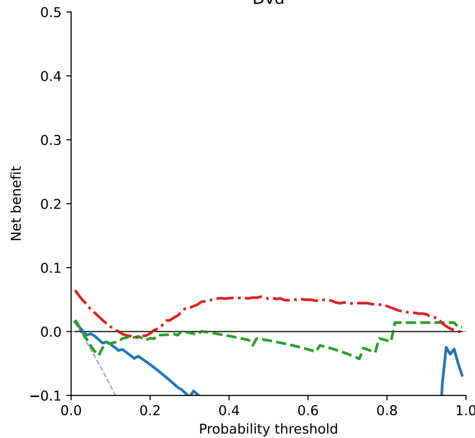
Dvd
