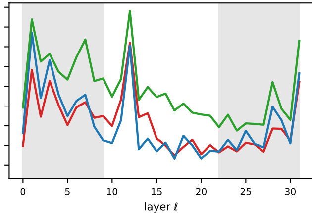
Llama-3.1-8B 4K
