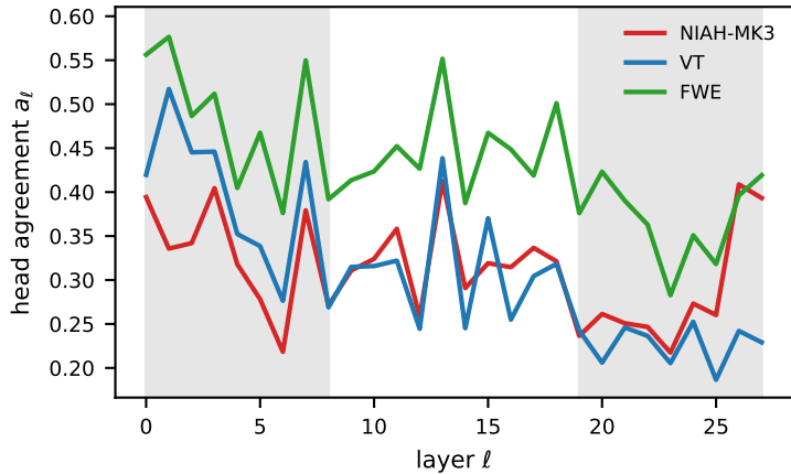
Qwen2.5-1.5B 4K
