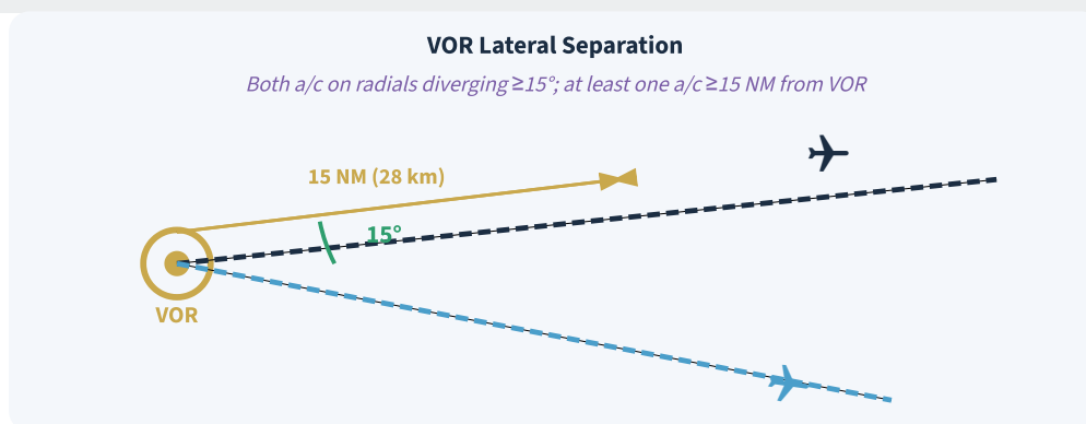
Fig 3.2 – VOR Lateral Separation ( 15^\circ divergence, 15 NM)
