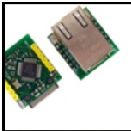
W5500 MINI MODULE SKU:- HW-884
