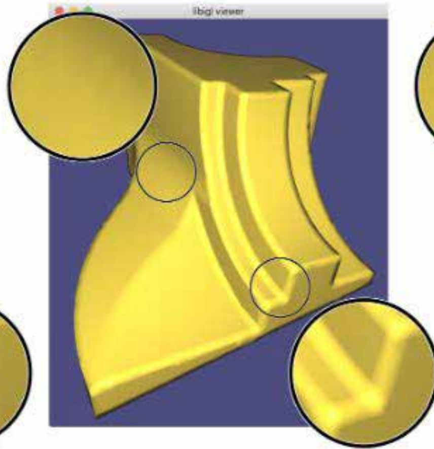
Per-Vertex Normals
