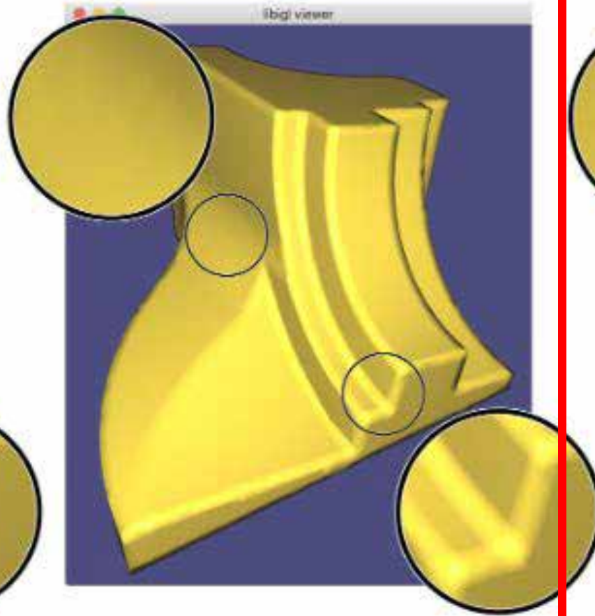
Per-Vertex Normals
