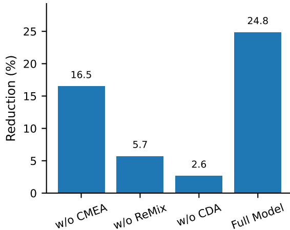
BRISQUE
