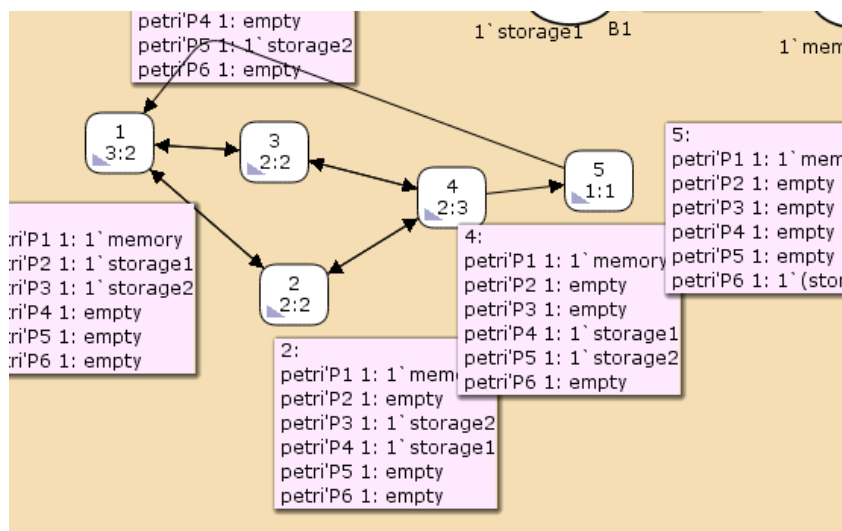
Figure 0.6: Граф пространства состояний
