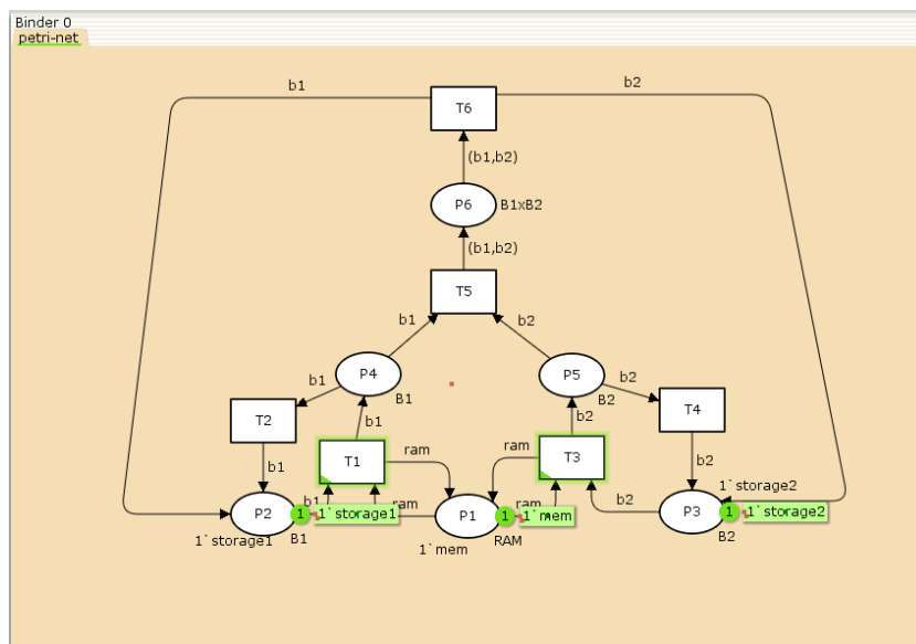
Figure 0.3: Модель задачи в CPN Tools
