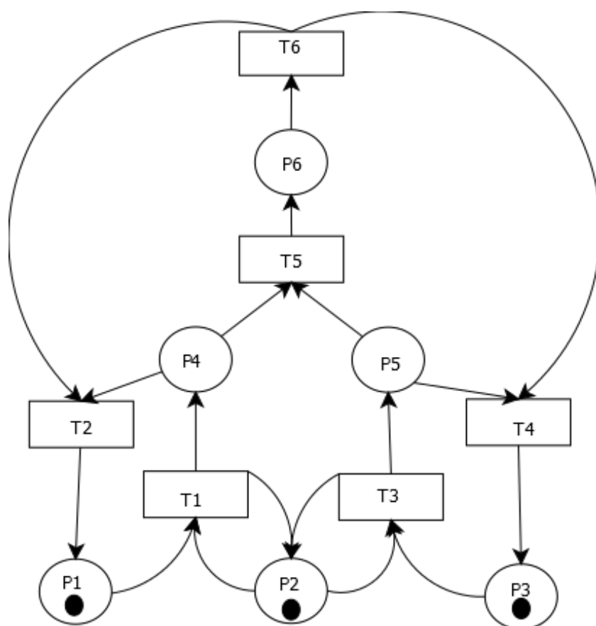
Figure 0.1: Сеть для выполнения домашнего задания
