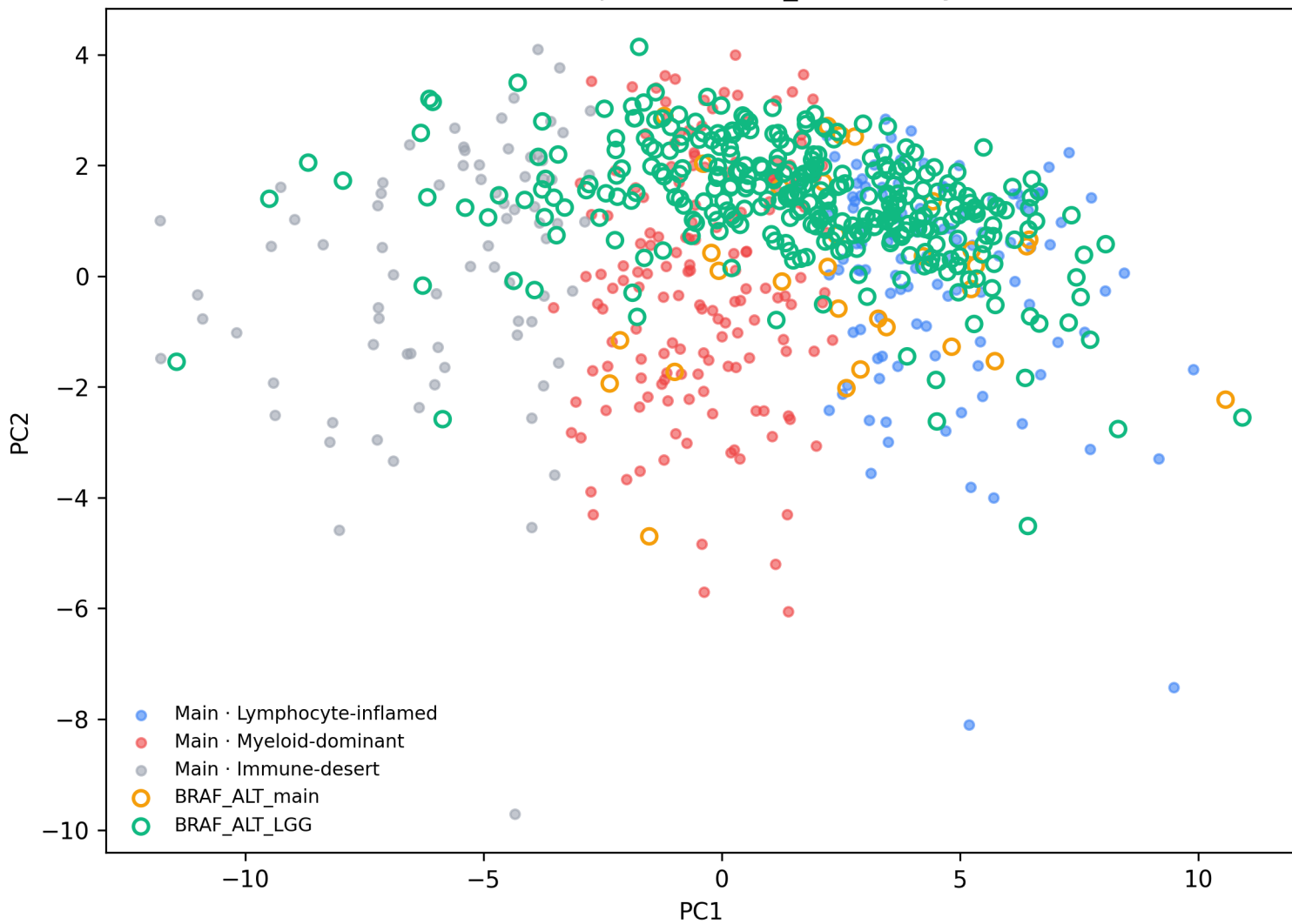
Main PCA space — BRAF_ALT overlay
