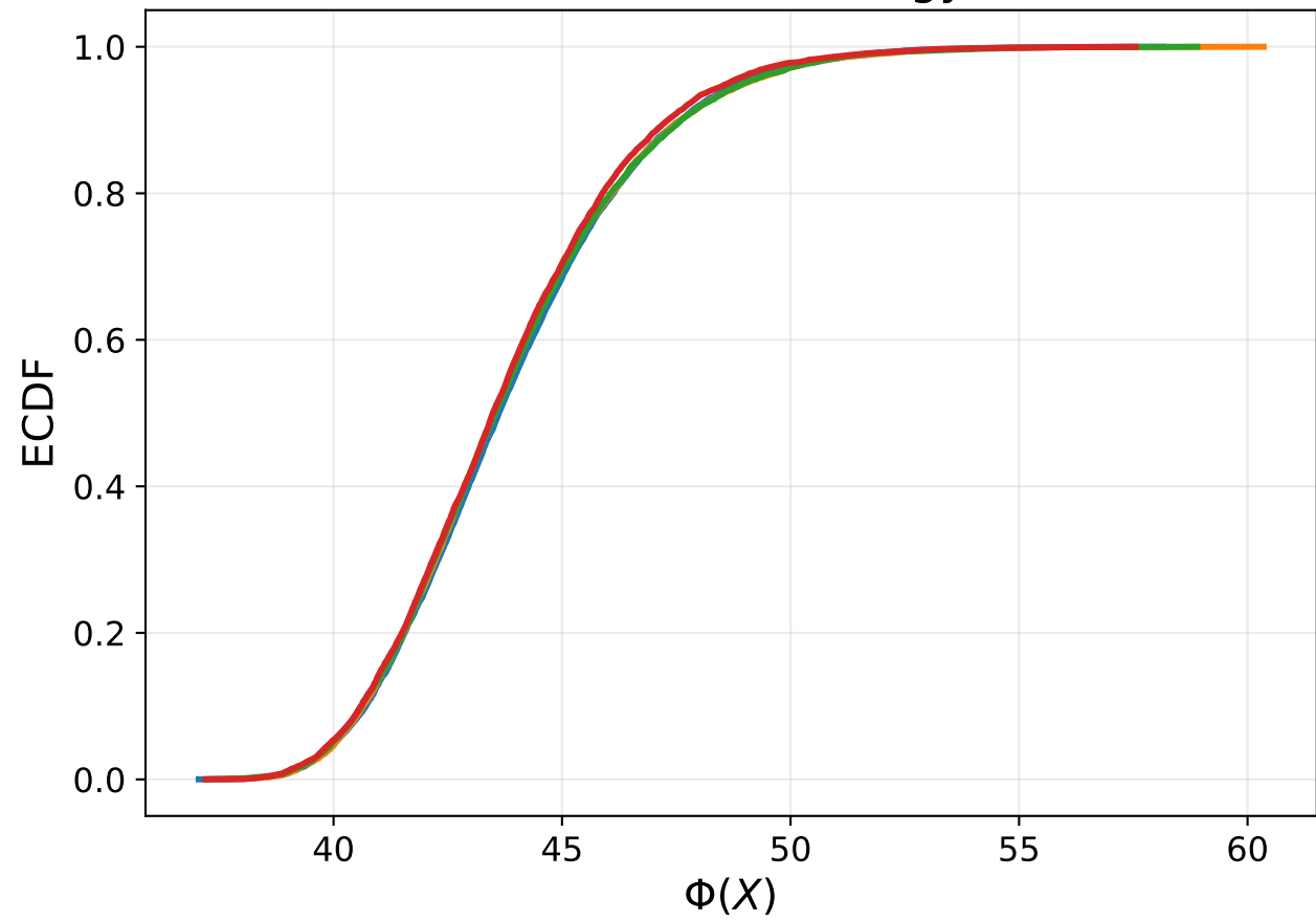
(b) Posterior energy
