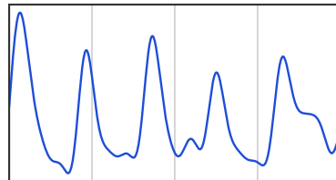
BIDMC
