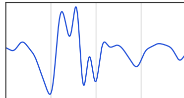
WESAD
