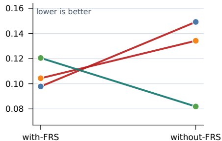
ECE
